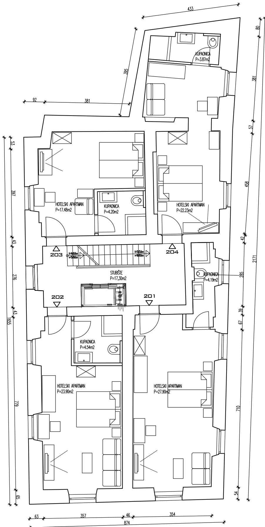
TLOCRT 2.KATA
