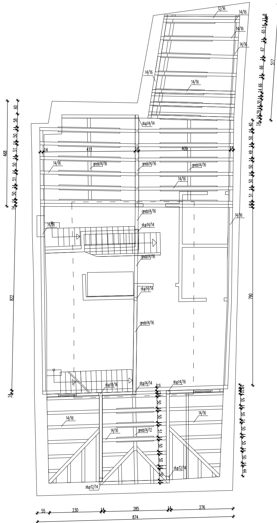
TLOCRT KROVIŠTA 4.KATA
