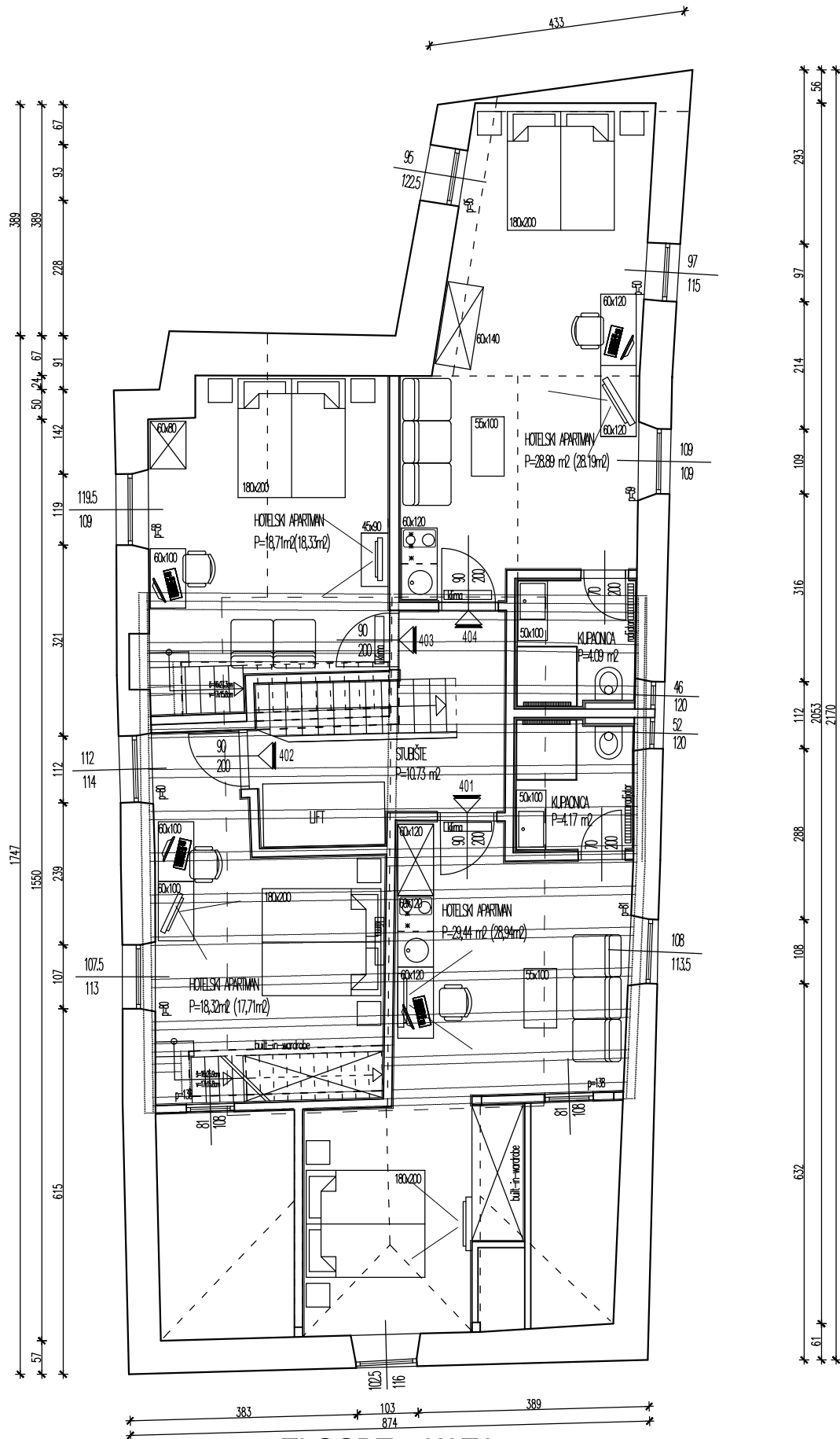
TLOCRT 4.KATA
