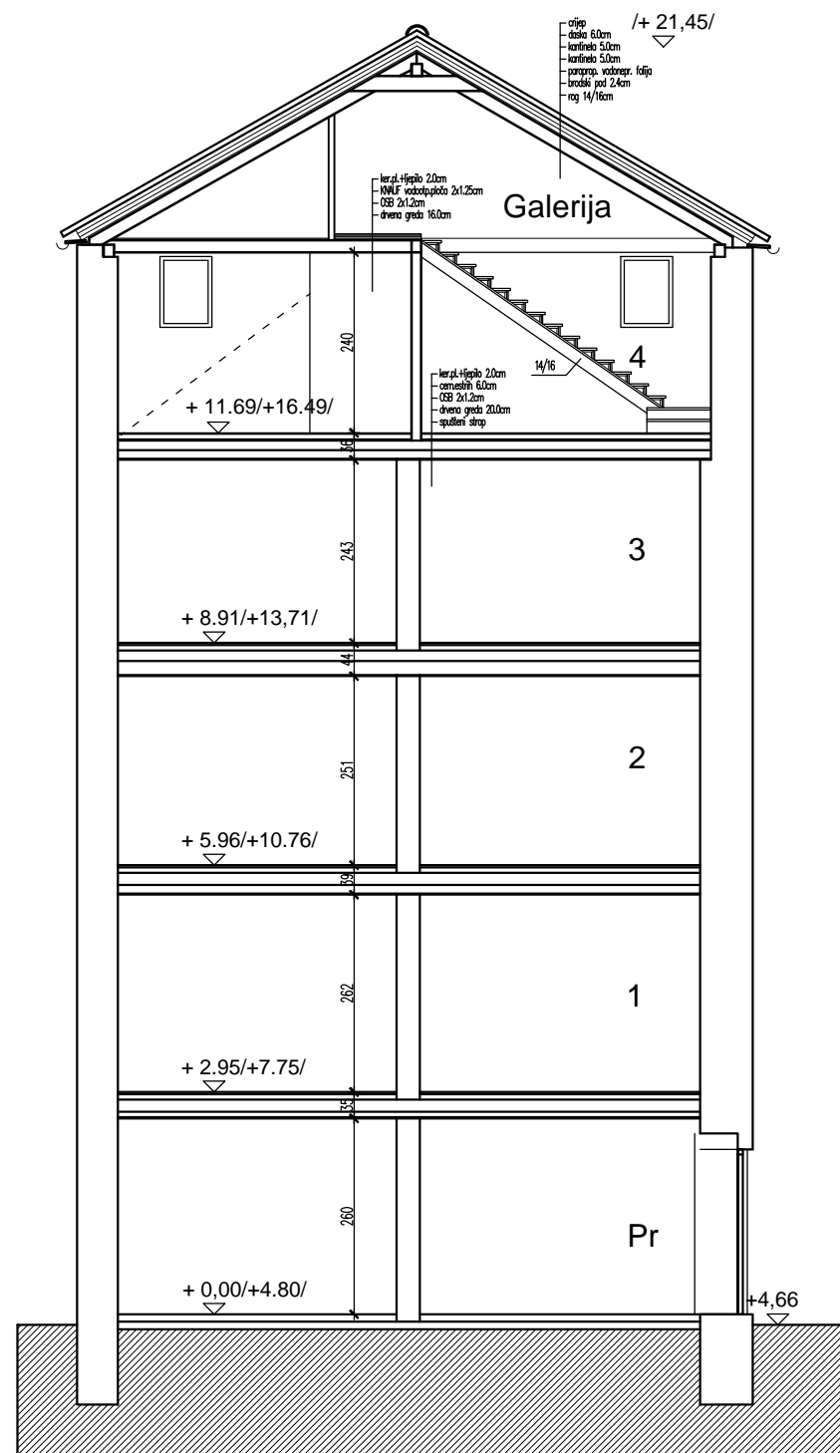
PRESJEK A-A
