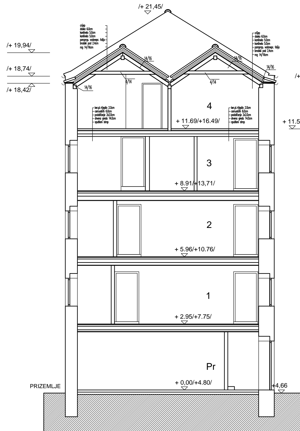
PRESJEK B-B
