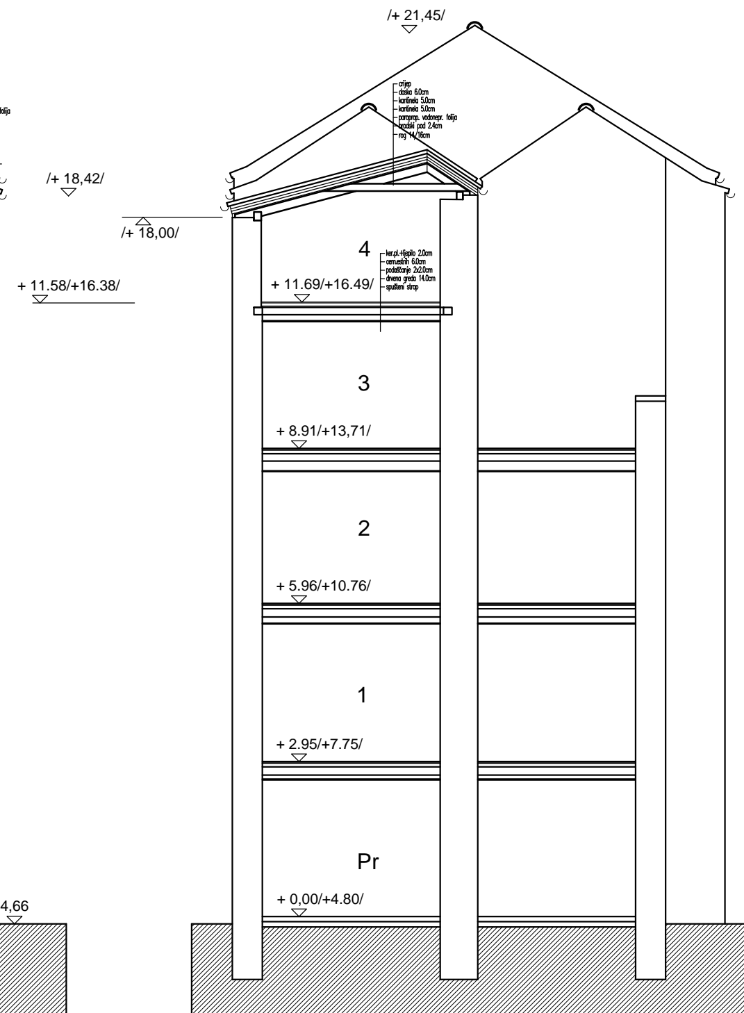
PRESJEK C-C
