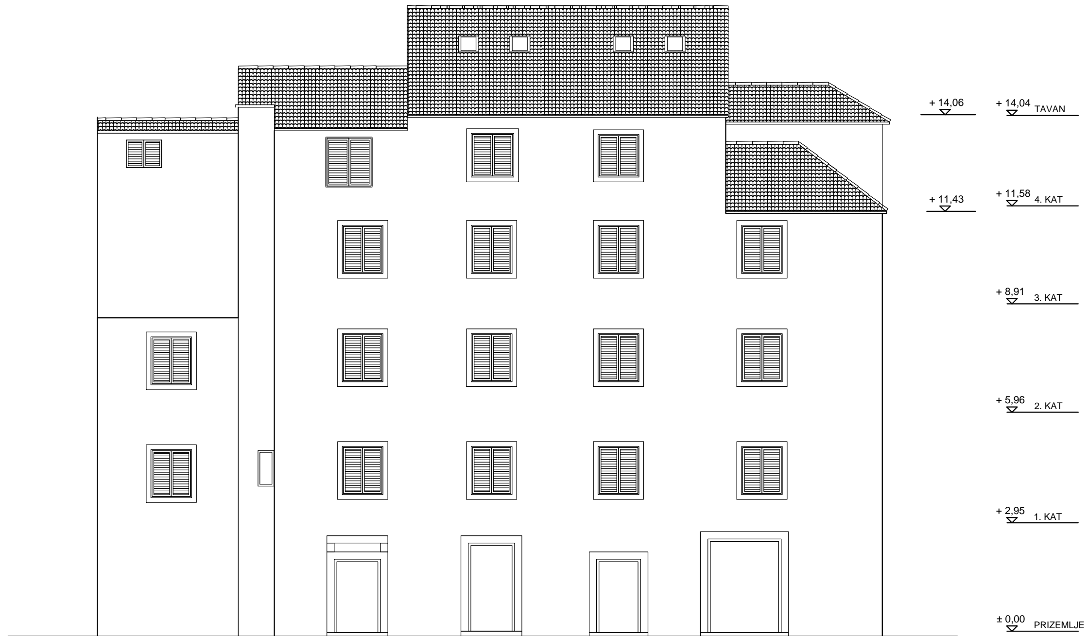
ZAPADNO PROČELJE
